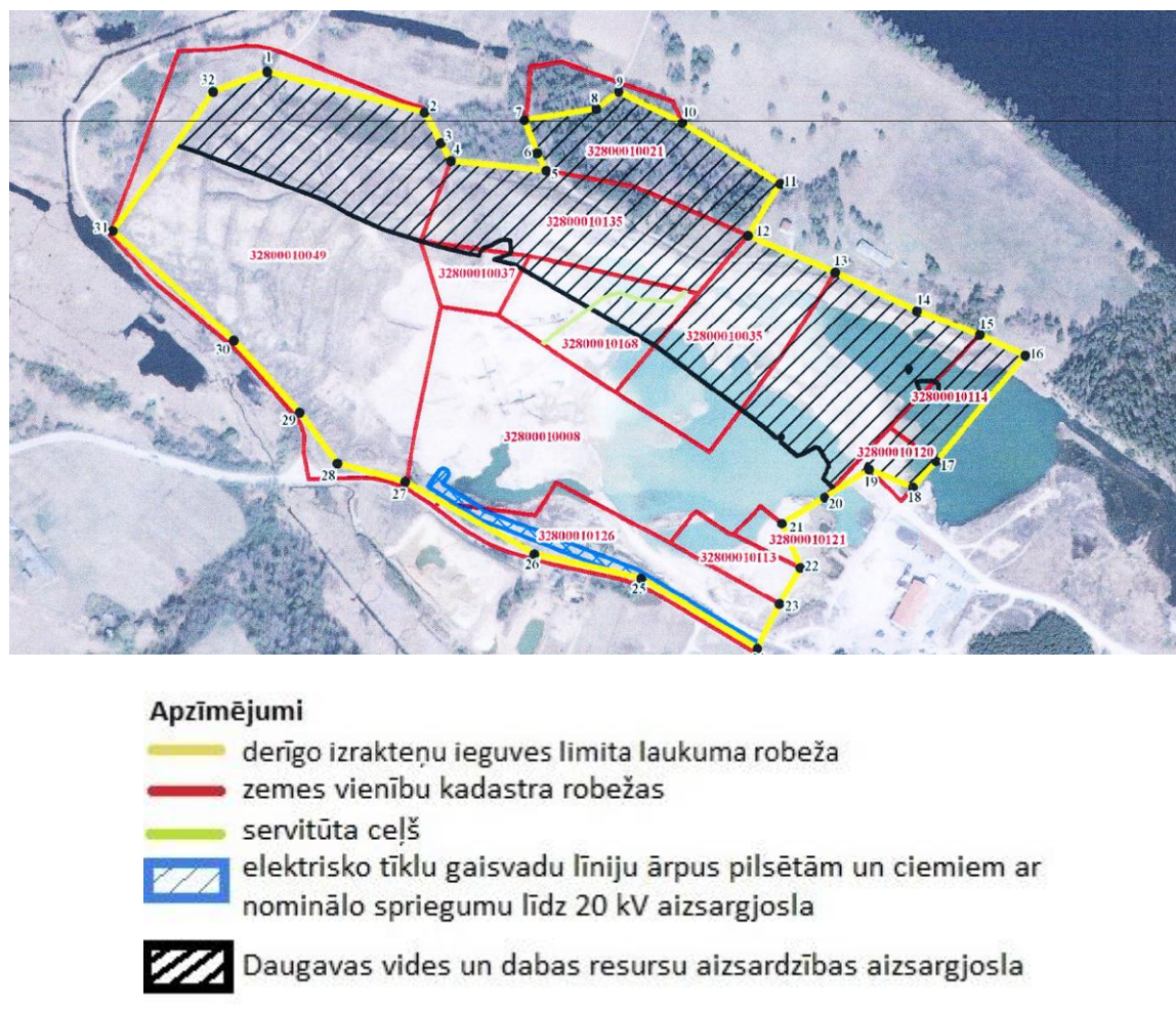
5.3.attēls. Aizsargjoslu izvietojums atradnē. (Avots: Derīgo izrakteņu ieguves limits, izsniedzējs VVD, 2018. gada 27. jūnijs.)
